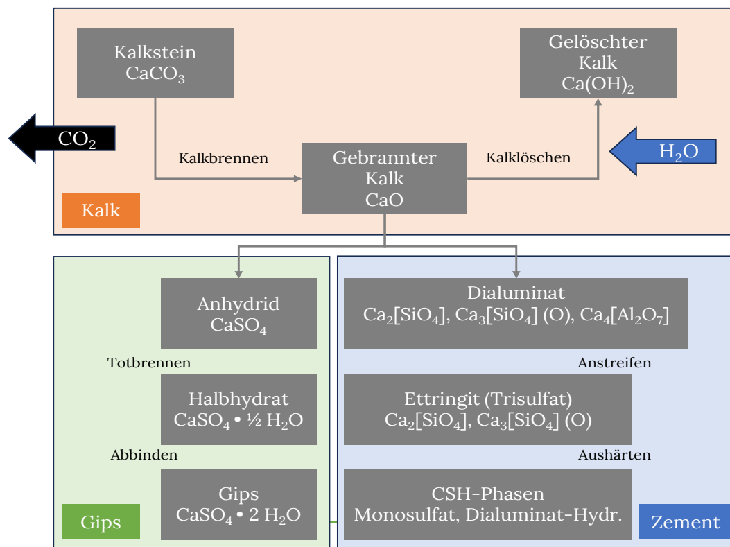
Abbildung 1: Schema zur Kalk-, Zement- und Gipsherstellung [Uni Freiburg 2002; Darstellung: Gansler/EMMD]
